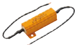
Load Resistor (50 x 15 x 15 mm) B111647 : 24V B112640 : 12V
